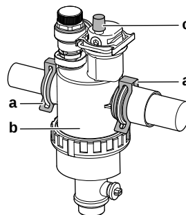
a Fermer b Filtre magnétique/pot de décantation c Vanne de purge d'air
