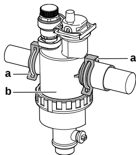
a Fermer b Filtre magnétique/pot de décantation
