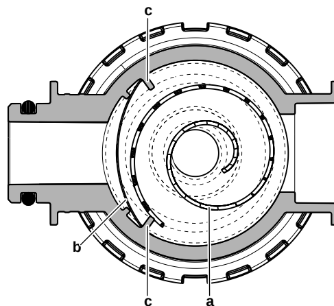
a Filtre enroulé b Filtre c Saillie
