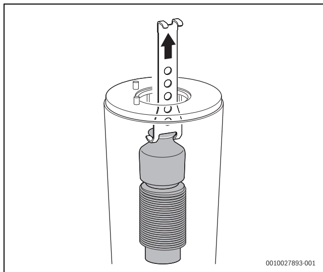
Fig. 49 Retirer le déflecteur supérieur
