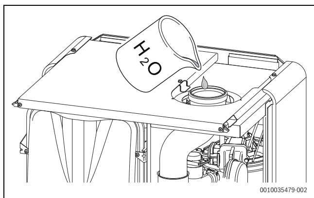
Fig. 26 Remplir le siphon des condensats avec de l'eau
