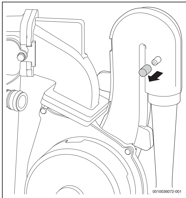
Fig. 42 Raccord de mesure sur le dispositif de mélange
