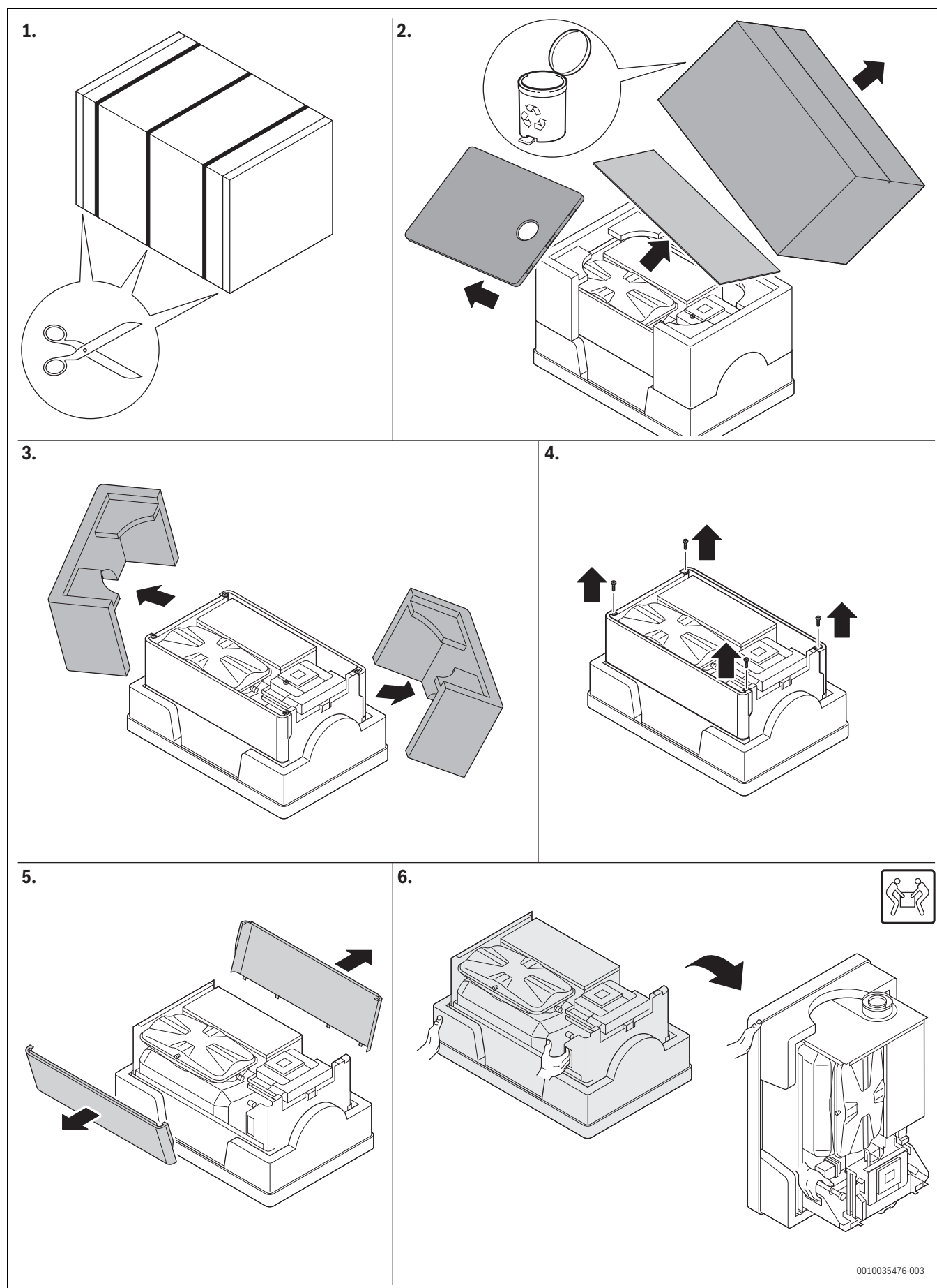
Fig. 20 Instructions de déballage
