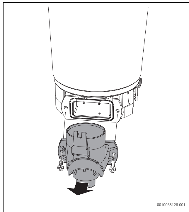
Fig. 54 Ouvrir la trappe de visite
