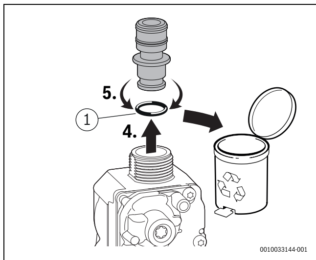
Fig. 65 Retrait de l'orifice
