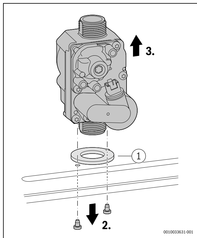
Fig. 67 Démontage du bloc gaz
