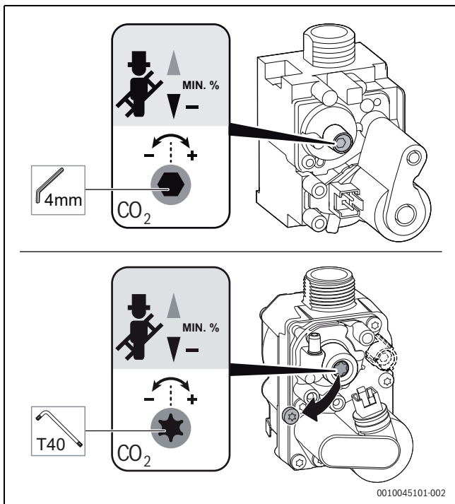
Fig. 40 Régler la teneur en \text{CO}_2/\text{O}_2 sur la puissance thermique nominale minimale
