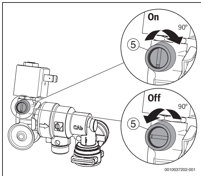
Fig. 29 Remplissage manuel avec le dispositif de remplissage automatique (accessoire)
