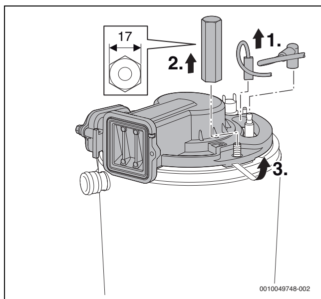
Fig. 46 Détacher le couvercle du brûleur
