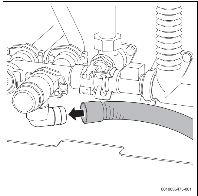
Fig. 23 Montage du tube sur la soupape de sécurité (circuit ECS)
