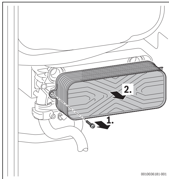
Fig. 43 Démontage de l'échangeur à plaques
