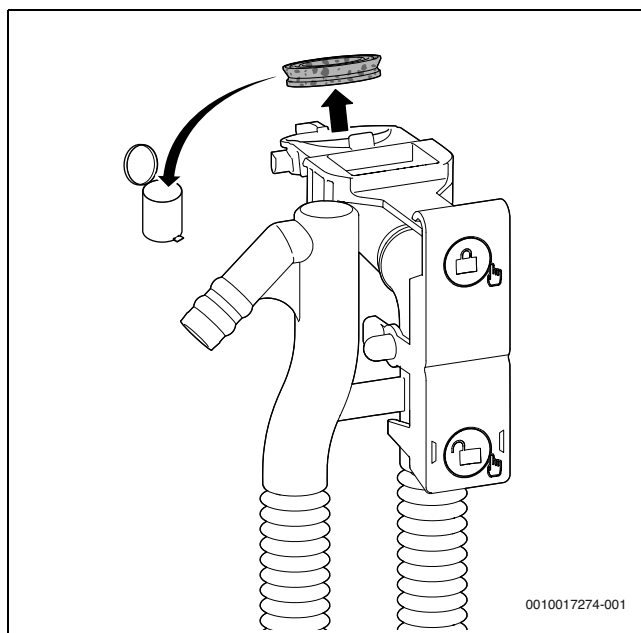
Fig. 58 Retrait du joint en haut sur le siphon de condensats
