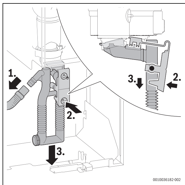
Fig. 56 Démonter le siphon des condensats
