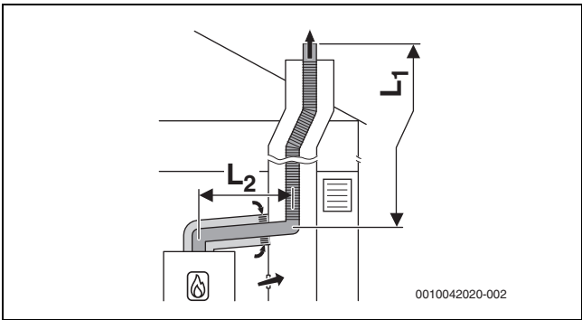
Fig. 12 Evacuation des fumées flexible dans le conduit selon B 53P avec arrivée d'air dépendant de l'air ambiant par le circuit d'air et de fumées concentrique dans le local d'installation
