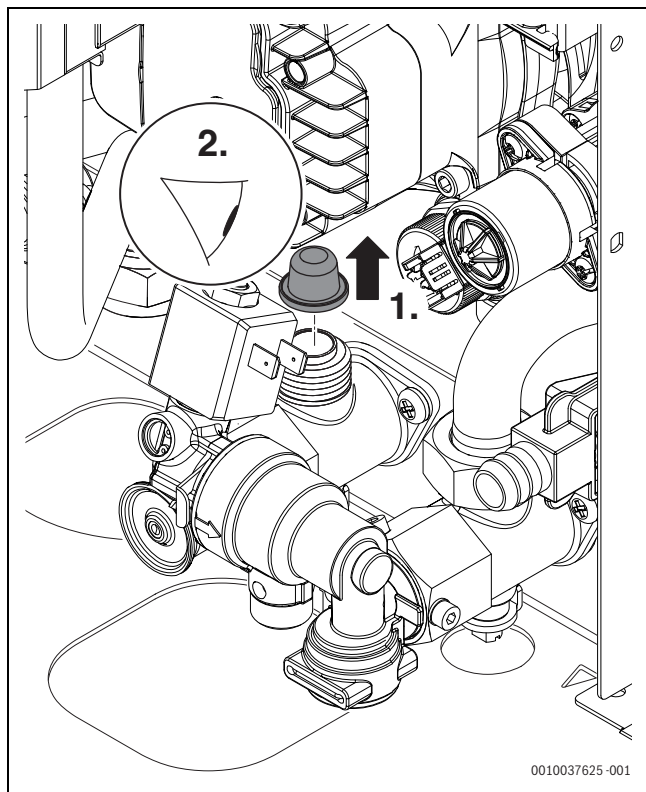
Fig. 63 Vérifier l'encrassement du filtre
