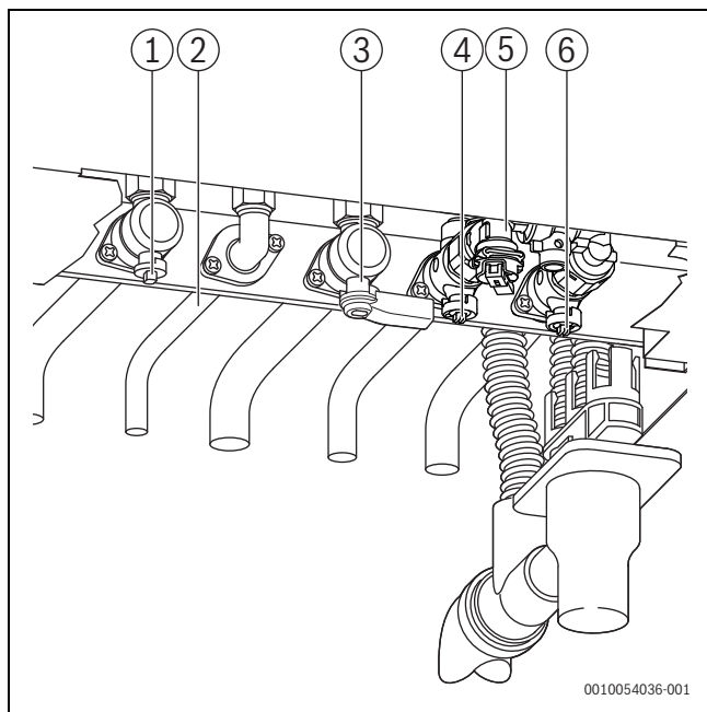
Fig. 28 Raccordements côté gaz et eau
