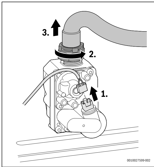
Fig. 64 Retrait du connecteur du bloc gaz et de l'écrou avec le tuyau du gaz
