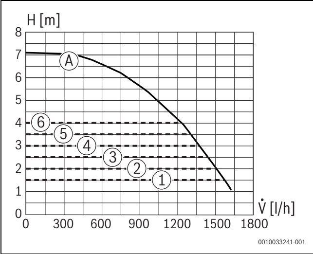
Fig. 76 Diagrammes de pompe et courbes caractéristiques de pompe
