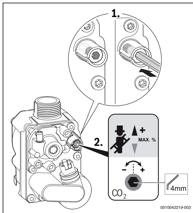
Fig. 39 CO 2 /O 2 -Régler la teneur en CO 2 /O 2 sur la puissance thermique nominale maximale, vanne gaz ajustable
