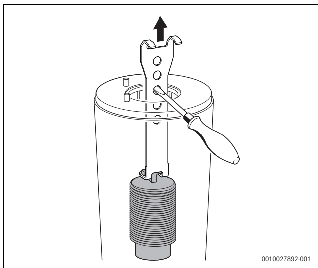
Fig. 50 Retirer le déflecteur inférieur
