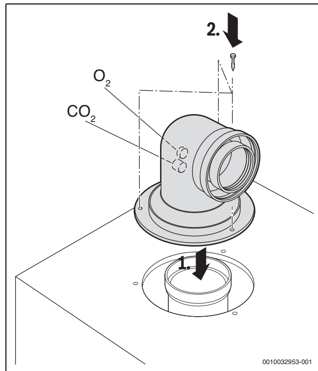
Fig. 27 Insérer les accessoires de fumisterie et fixer avec trois vis.
