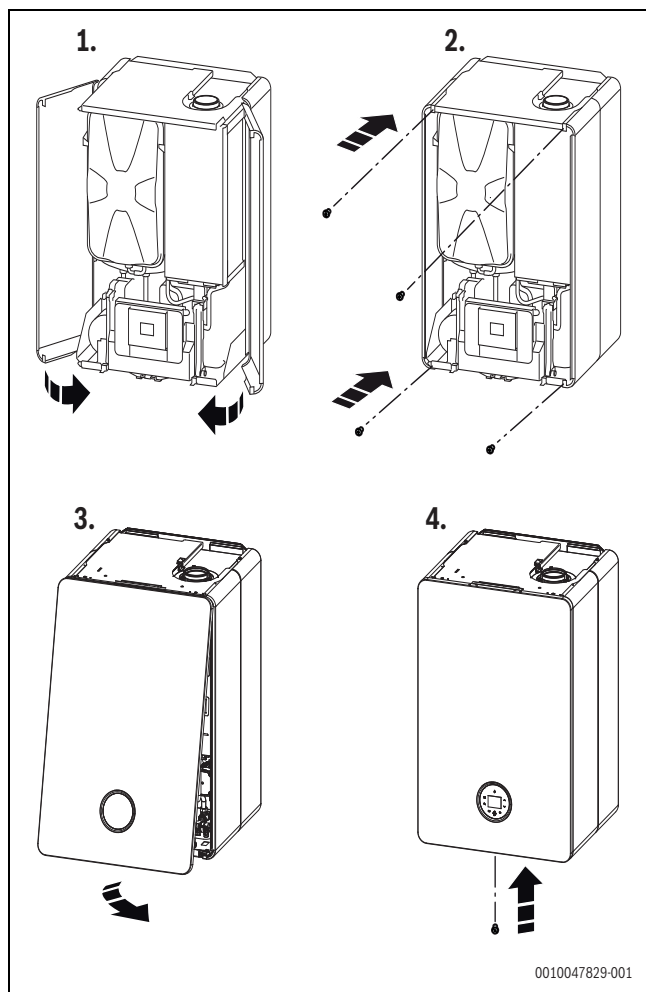
Fig. 33 Montage du carénage
