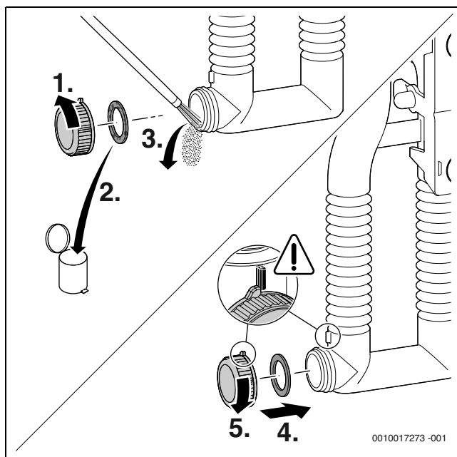
Fig. 57 Nettoyage du siphon de condensats
