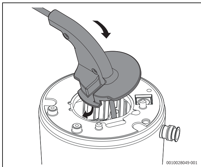
Fig. 51 Insertion de la brosse dans le corps de chauffe
