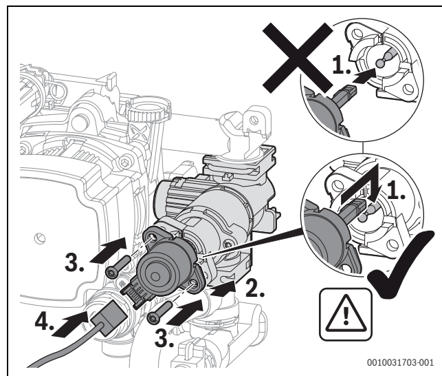
Fig. 75 Remonter le moteur au niveau de la vanne 3 voies (variante avec vis)
