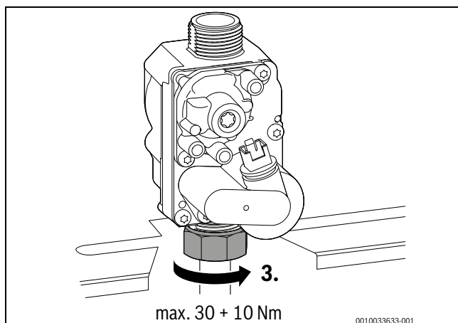
Fig. 69 Respect du couple de serrage
