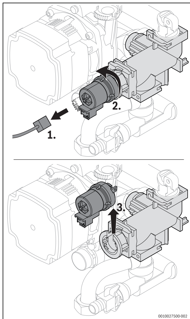
Fig. 72 Démontez le moteur au niveau de la vanne 3 voies (variante sans vis)
