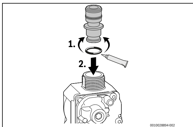
Fig. 70 Insertion l'orifice de réglage de gaz
