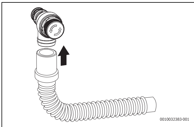
Fig. 22 Montage du tube sur la soupape de sécurité (chauffage)
