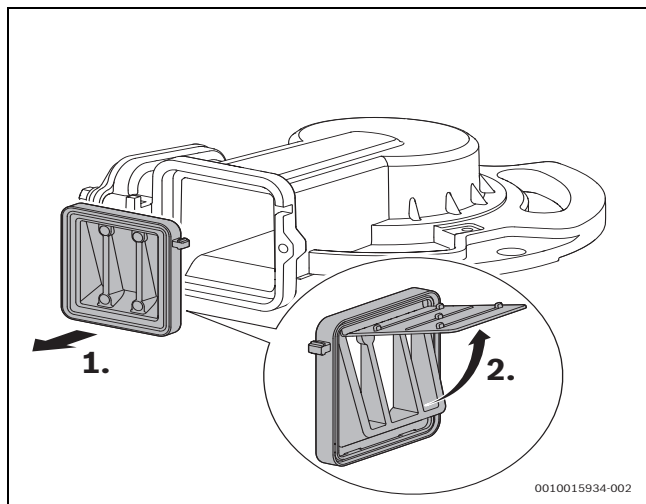
Fig. 47 Clapet anti-retour du dispositif de mélange
