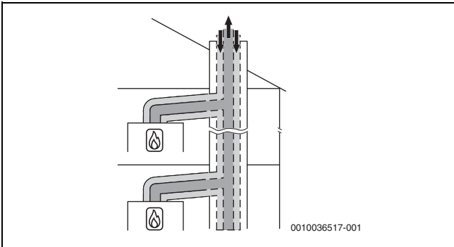
Fig. 13 Raccordement de plusieurs foyers selon C 43P avec circuit d'air et de fumées concentrique dans le local d'installation
