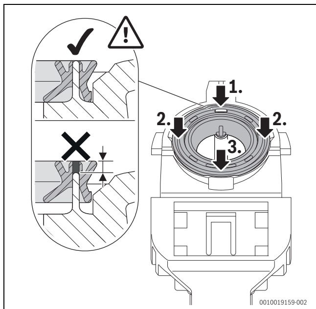
Fig. 60 Appui sur le joint
