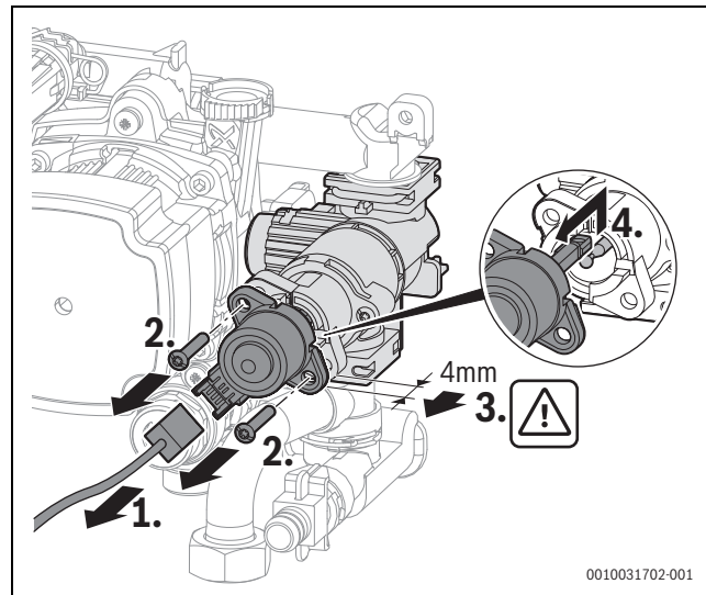
Fig. 74 Démontez le moteur au niveau de la vanne 3 voies (variante avec vis)
