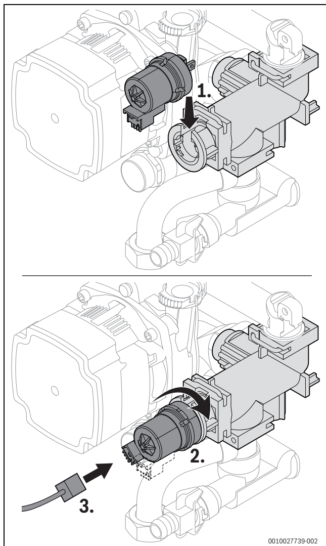
Fig. 73 Remonter le moteur au niveau de la vanne 3 voies (variante sans vis)
