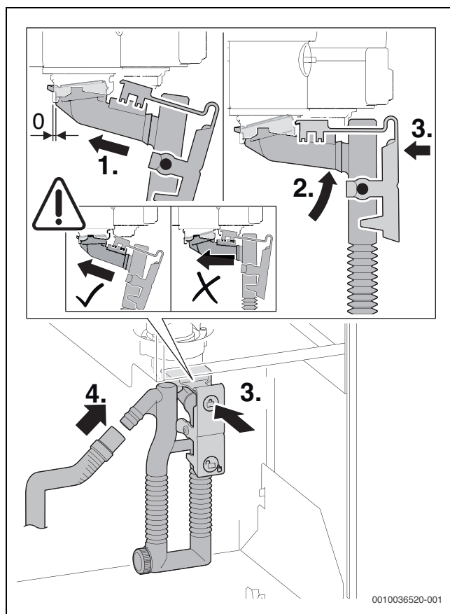
Fig. 61 Insertion du siphon de condensats
