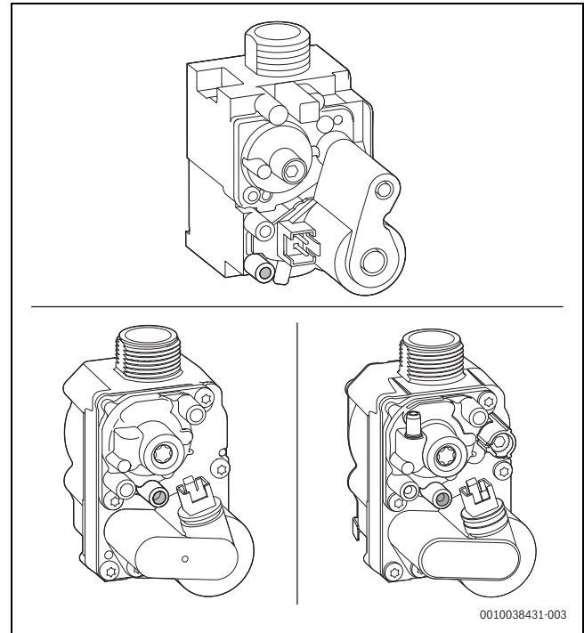
Fig. 35 En haut et en bas à gauche: vanne gaz fixe, en bas à droite: vanne gaz ajustable
