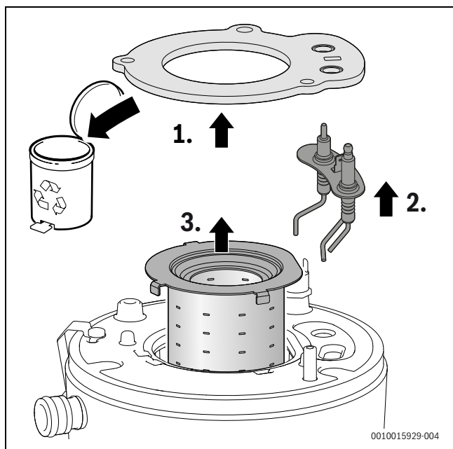
Fig. 48 Retirer le brûleur
