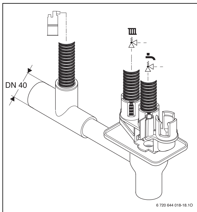
Fig. 25 Monter le tuyau des condensats et les flexibles des soupapes de sécurité sur le siphon
