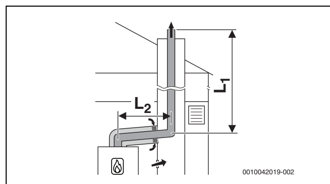
Fig. 11 Évacuation des fumées rigide dans le conduit selon B 53p avec arrivée d'air dépendant de l'air ambiant par le circuit d'air et de fumées concentrique dans le local d'installation
