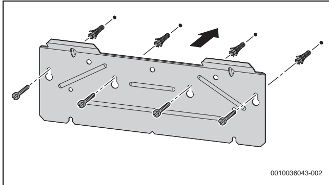
Fig. 21 Montage de la traverse d'accrochage
