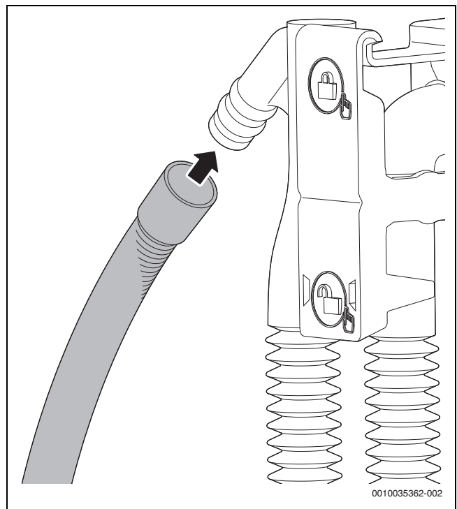
Fig. 24 Monter le tuyau des condensats sur le siphon de condensats.
