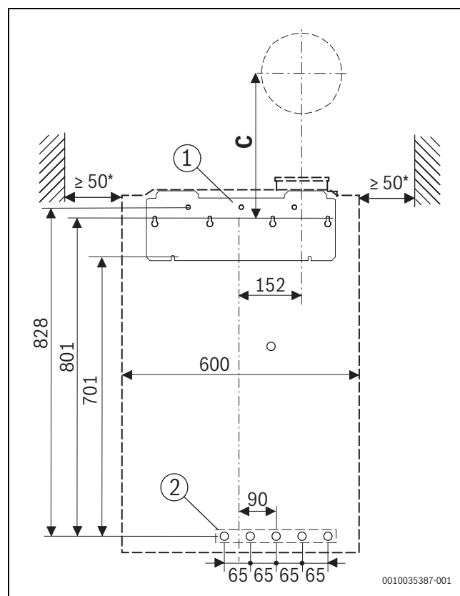
Fig. 3 Vue avant (mm)
