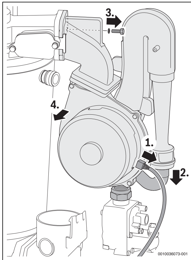
Fig. 45 Démontage du ventilateur avec le dispositif de mélange
