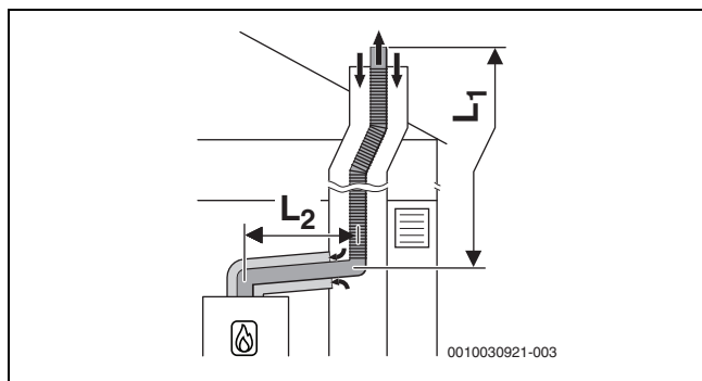
Fig. 10 Evacuation des fumées flexible selon C 93x dans le conduit et circuit d'air et de fumées concentrique dans le local d'installation
