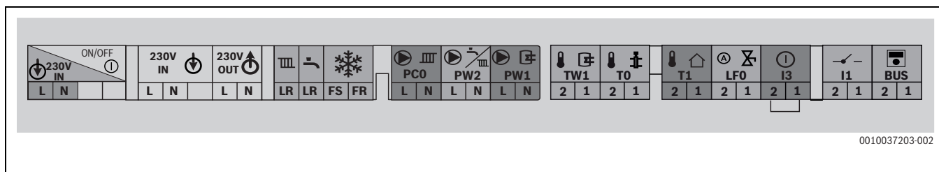
Fig. 32 Bornier pour accessoires externes
