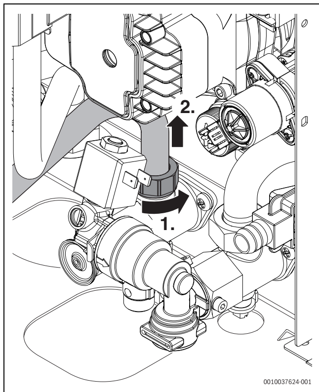
Fig. 62 Retirer le tuyau au raccord d'entrée eau froide
