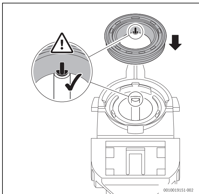
Fig. 59 Alignement du nouveau joint sur le siphon de condensats
