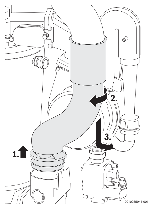
Fig. 44 Démontez le tuyau de fumée
