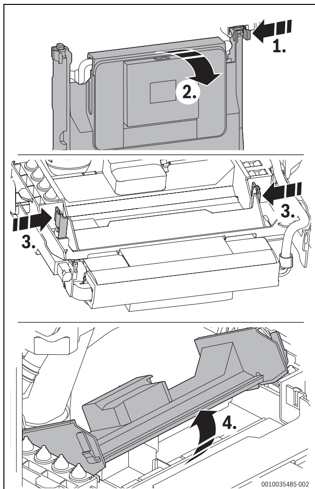
Fig. 30 Ouvrir l'appareil de commande
