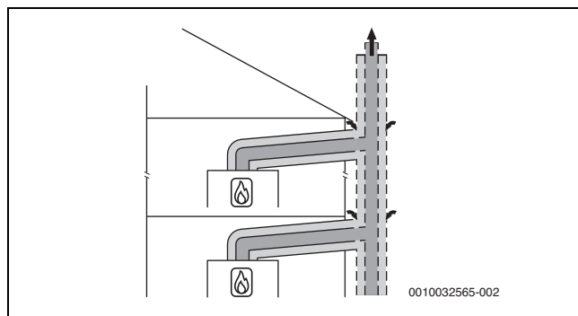
Fig. 15 Raccordement de plusieurs foyers selon C_{(12)3x} avec circuit d'air et de fumées concentrique dans le local d'installation
