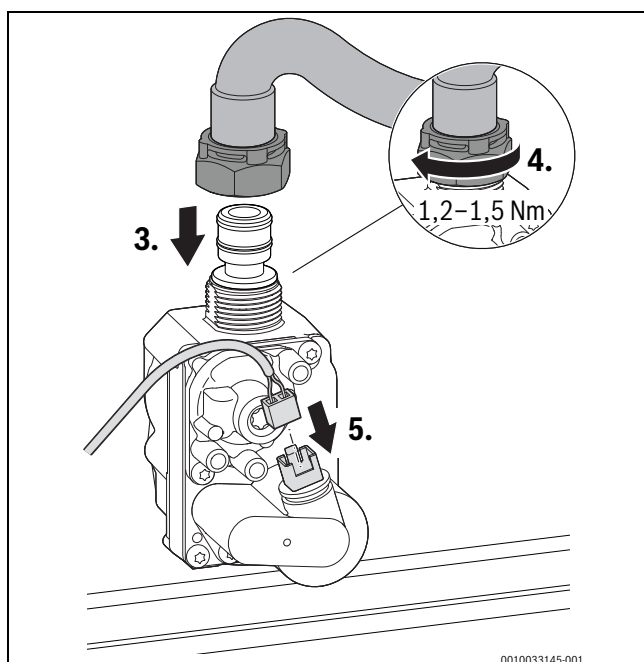
Fig. 71 Raccordement du tuyau du gaz et du connecteur – Respect du couple de serrage
