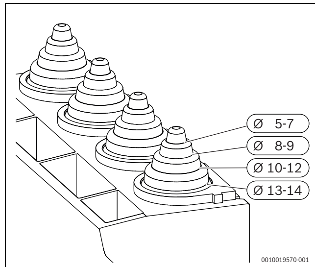
Fig. 31 Adaptation du serre-câbles au diamètre du câble
