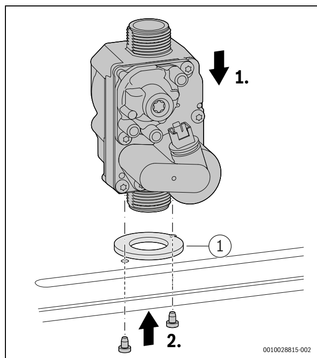
Fig. 68 Installation du bloc gaz
