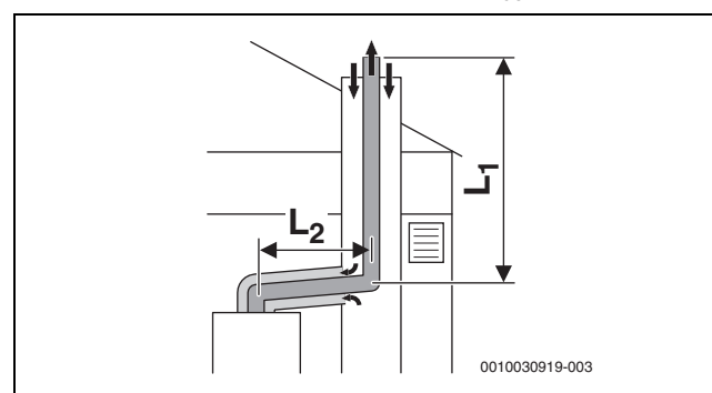
Fig. 9 Evacuation des fumées rigide selon C 93x dans le conduit et circuit d'air et de fumées concentrique dans le local d'installation
