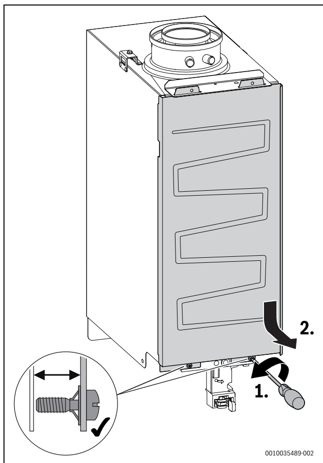
Fig. 36 Retirer le capot du brûleur
