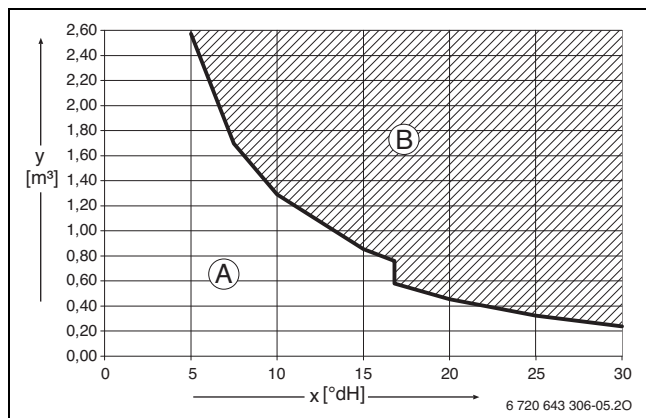
Fig. 17 Conditions requises pour l'eau de remplissage et d'appoint en °dH sur les appareils < 50 kW
