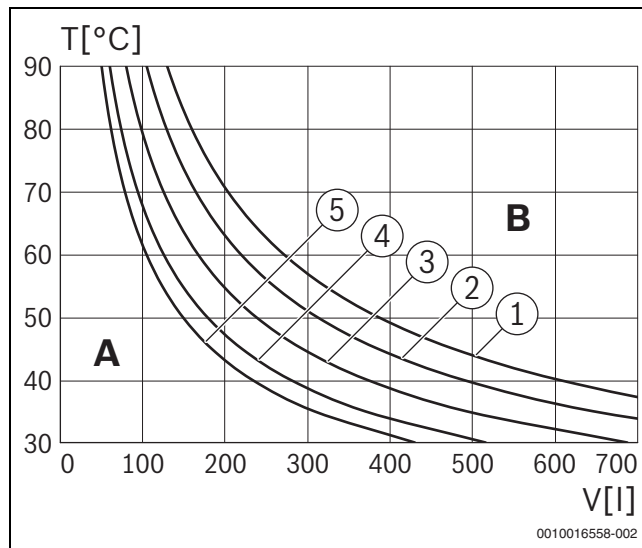
Fig. 19 Courbes caractéristiques du vase d'expansion
