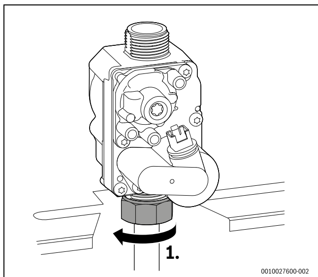
Fig. 66 Desserrage de l'écrou
