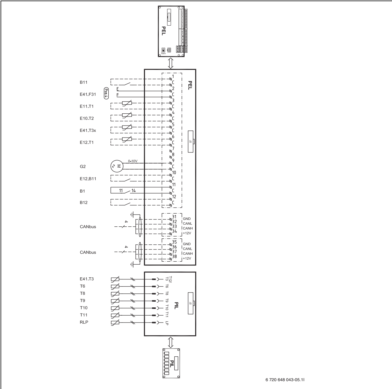
Fig. 27 Schéma électrique complets des raccordements (courant faible)
