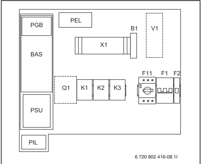
Fig. 22 Vue d'ensemble de la carte électronique
