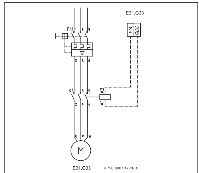
Fig. 29 Raccordement de la pompe à eau souterraine
