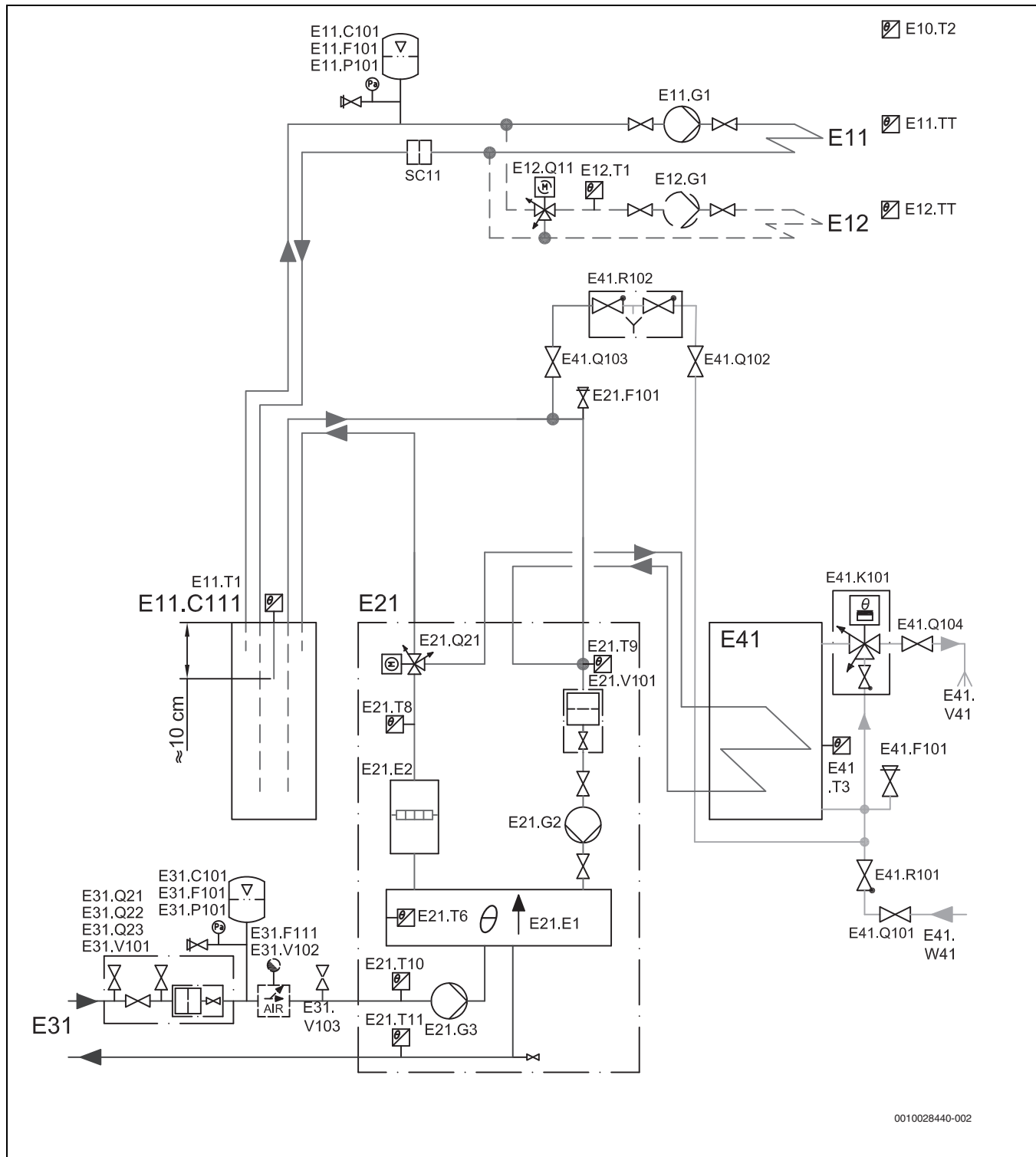
Fig. 8 Circuit de chauffage sans vanne mélangeuse avec réservoir de service et ballon d'eau chaude extérieur
