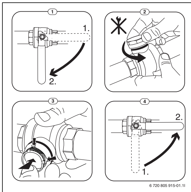
Fig. 46 Nettoyage du filtre
