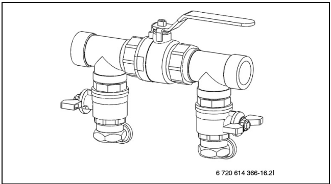
Fig. 15 Kit de remplissage
