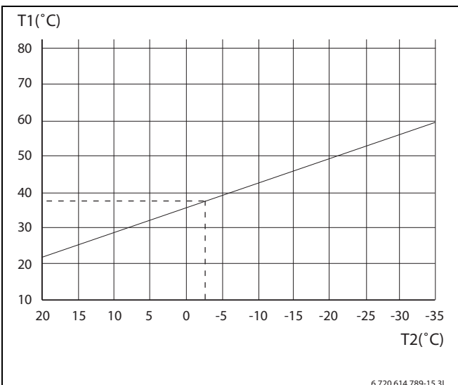
Fig. 36 Radiateur
