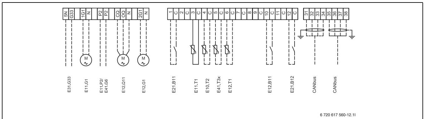
Fig. 28 Connexions externes
