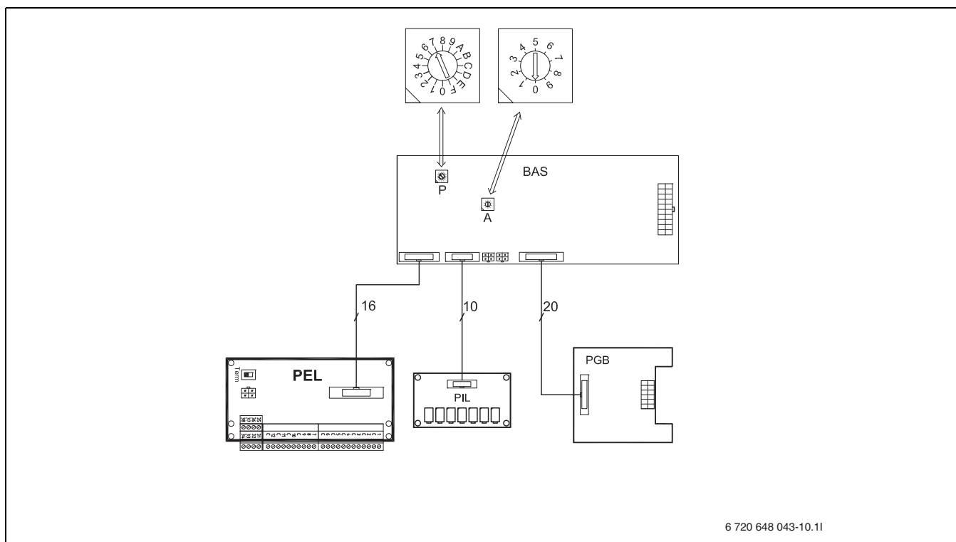
Fig. 24 Câblage de la carte électronique
