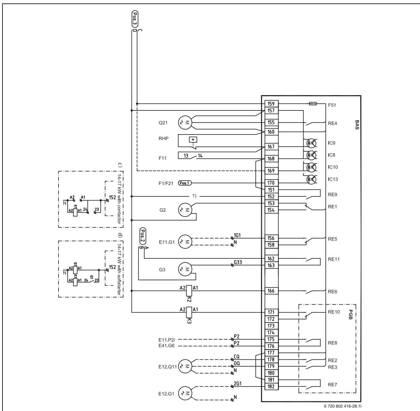
Fig. 26 Schéma électrique complets des raccordements (230V)
