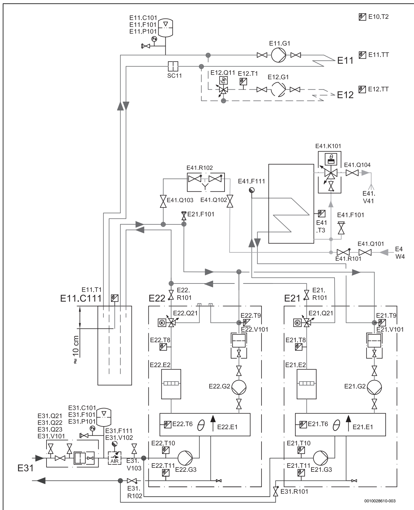
Fig. 9 Deux pompes à chaleur (raccordement en cascade) avec circuit de chauffage avec et sans vanne mélangeuse, réservoir de service et ballon d'eau chaude extérieur
