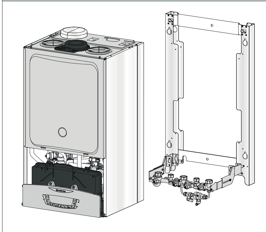
SCHÉMA 5 - REMPLACEMENT AVEC KIT BARRETTE 3319211 + CADRE ÉCARTEUR 3678416
