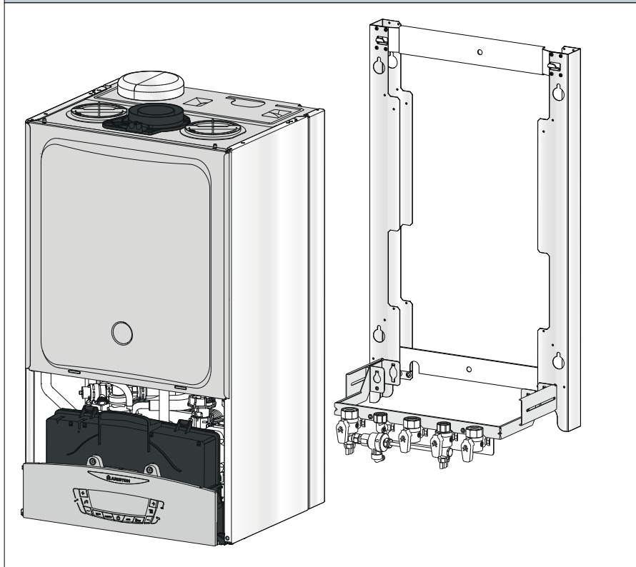
SCHÉMA 4 - REMPLACEMENT AVEC KIT BARRETTE 3319211 ET SANS CADRE ÉCARTEUR
