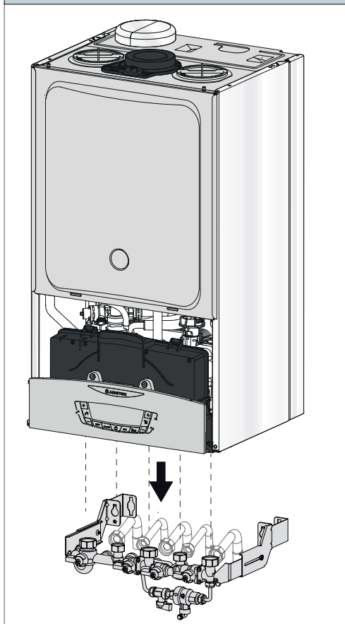
SCHÉMA 4 - REMPLACEMENT AVEC KIT BARRETTE 3319211 ET SANS CADRE ÉCARTEUR
