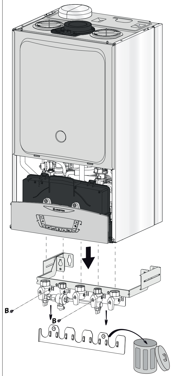
SCHÉMA 2 - INSTALLATION NEUVE SANS CADRE ÉCARTEUR - KIT BARRETTE 3319206
