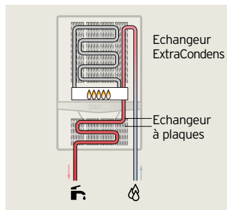
ECS préchauffée dans l'échangeur ExtraCondens avant son passage dans l'échangeur à plaques
