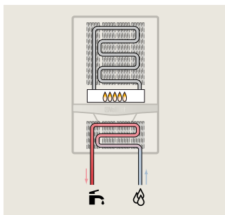
Eau chaude sanitaire (ECS) chauffée dans un échangeur à plaques dans une chaudière à condensation classique
